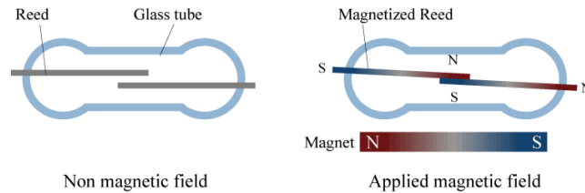
Imagen 2. Diagrama de funcionamiento del interruptor de láminas.
